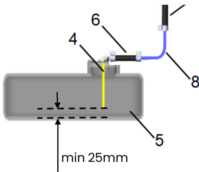
Rysunek 4. Odległość końca ujęcia paliwa od dna zbiornika.
