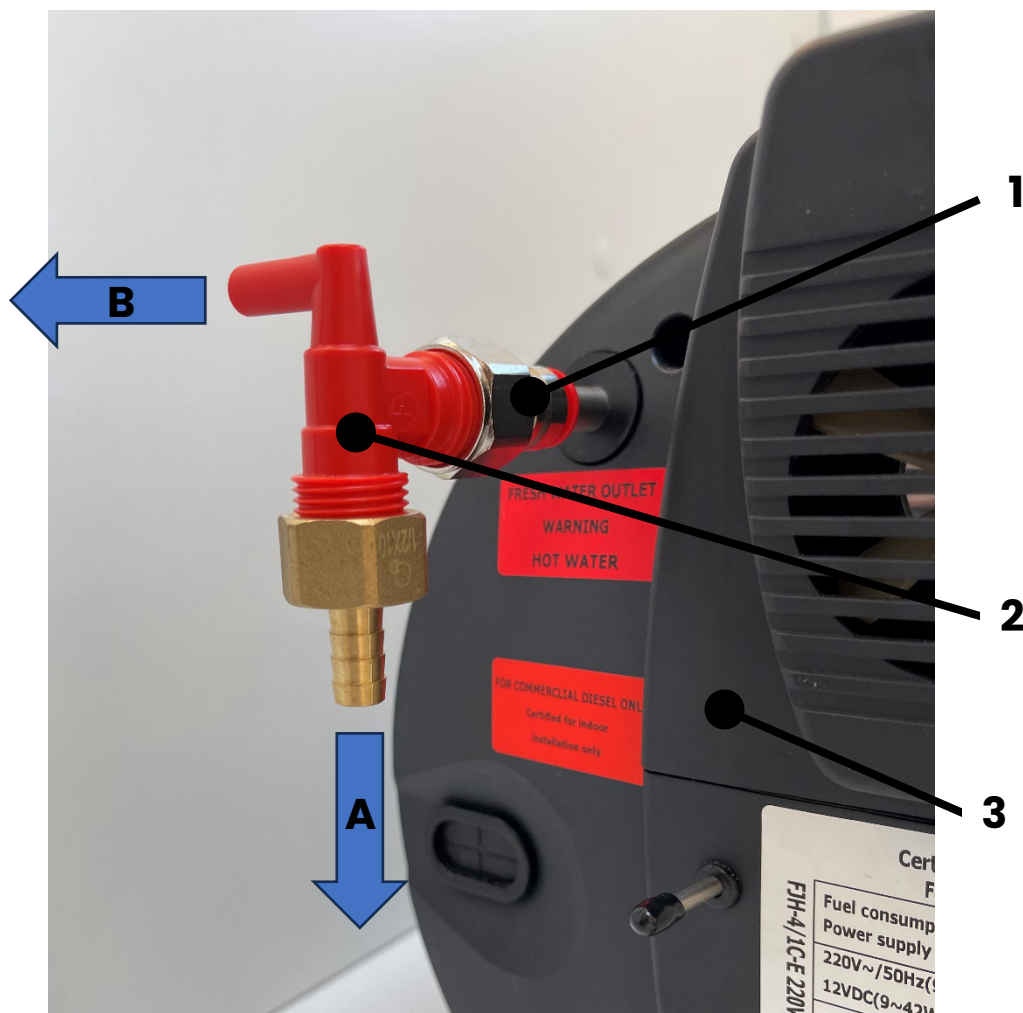
Rysunek 6. Podłączenie instalacji wodnej po stronie ciepłej.
