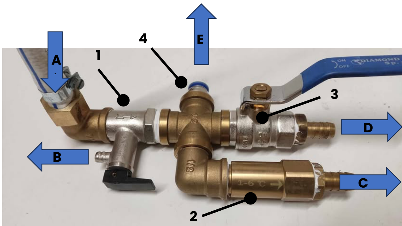
Rysunek 5. Podłączenie instalacji wodnej po stronie zimnej Bojlera Combi – Przykład.
