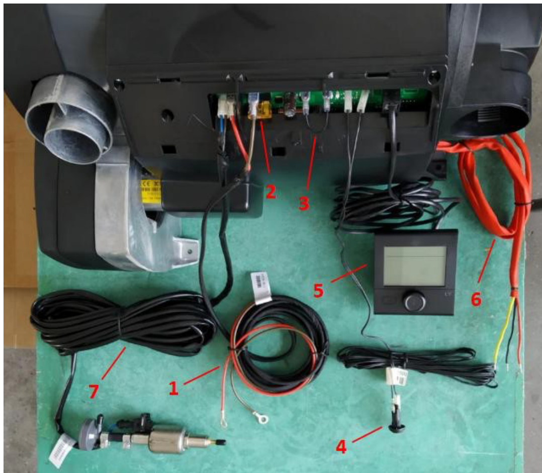
Rysunek 7 – Okablowanie.
