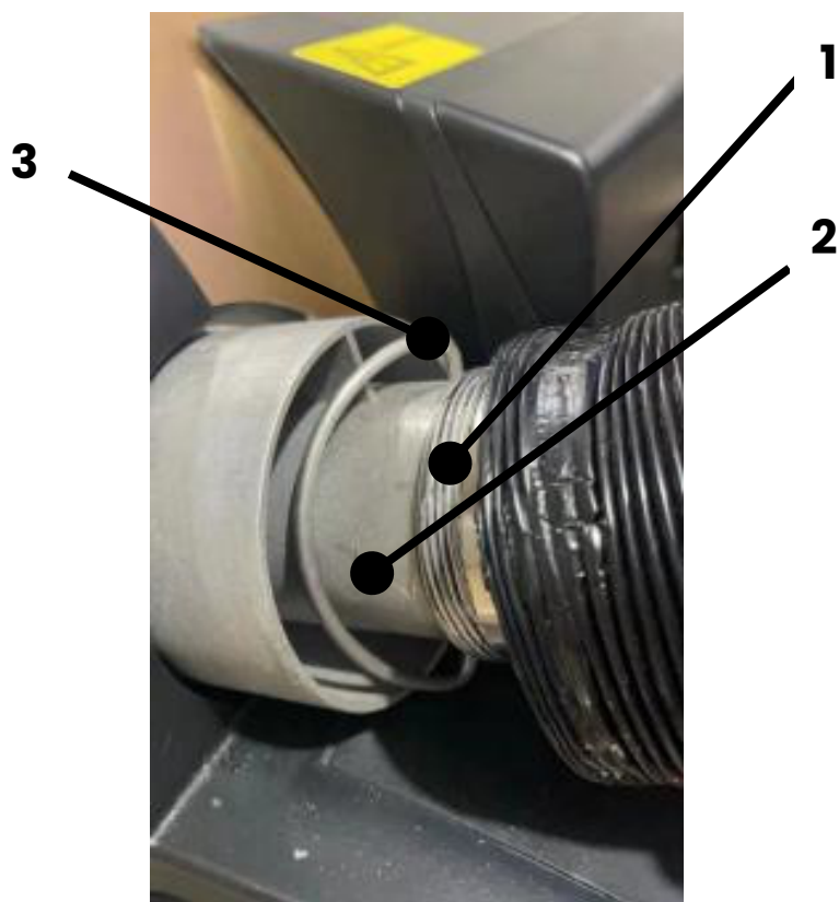
Rysunek 10. Podłączenie portu wydechowego JP Heater Combi. 1-Rura wydechowa (tłumik) 2-Port wydechowy, 3-Zatrzask sprężynowy.
