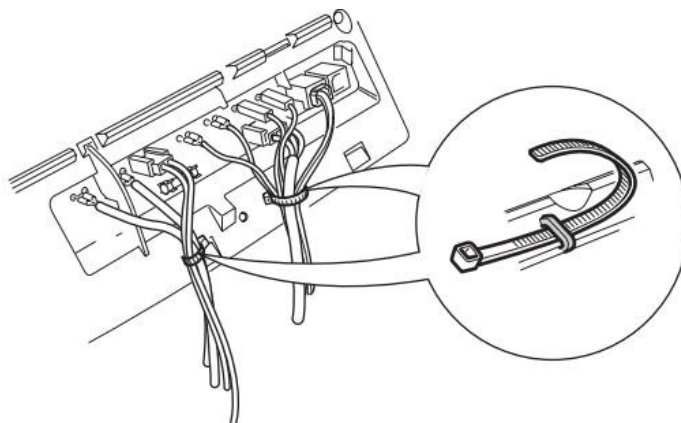
Rysunek 21 – Sposób zamocowania przewodów
