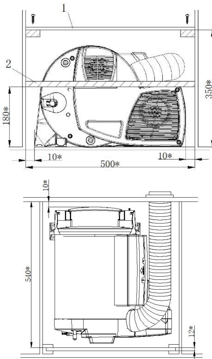
Rysunek 1 – minimalna przestrzeń montażowa
