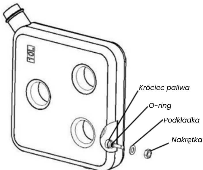
Rysunek 16 –Sposób montażu ujęcia paliwa w dodatkowym zbiorniku.
