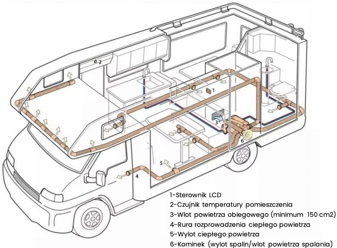
Rysunek 1- Typowa instalacja ogrzewacza Combi
