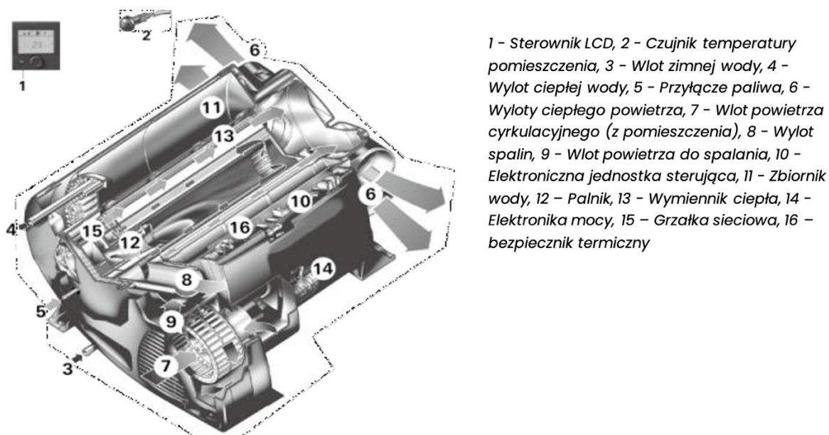
Rysunek 2 - Schemat ogrzewacza Combi
