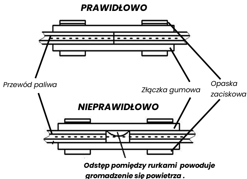
Rysunek 15.1 –Prawidłowe i nie prawidłowe połączenie przewodów linii paliwowej.
