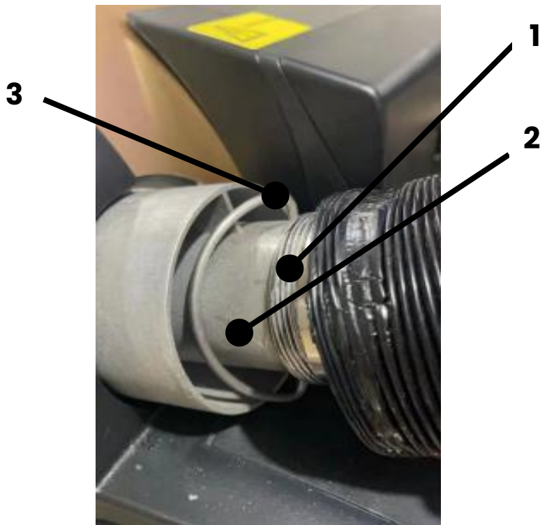
Rysunek 10. Podłączenie portu wydechowego JP Heater Combi. 1-Rura wydechowa (tłumik) 2-Port wydechowy, 3-Zatrzask sprężynowy.
