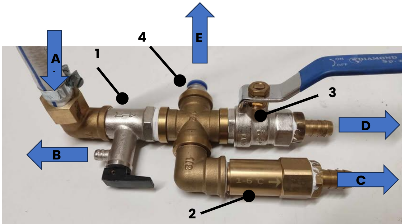
Rysunek 5. Podłączenie instalacji wodnej po stronie zimnej Bojlera Combi – Przykład.
