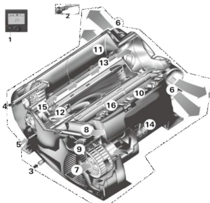
Rysunek 2 - Schemat ogrzewacza Combi
