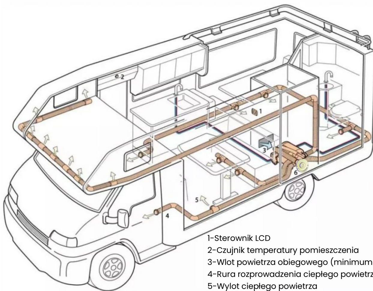
Rysunek 1- Typowa instalacja ogrzewacza Combi
