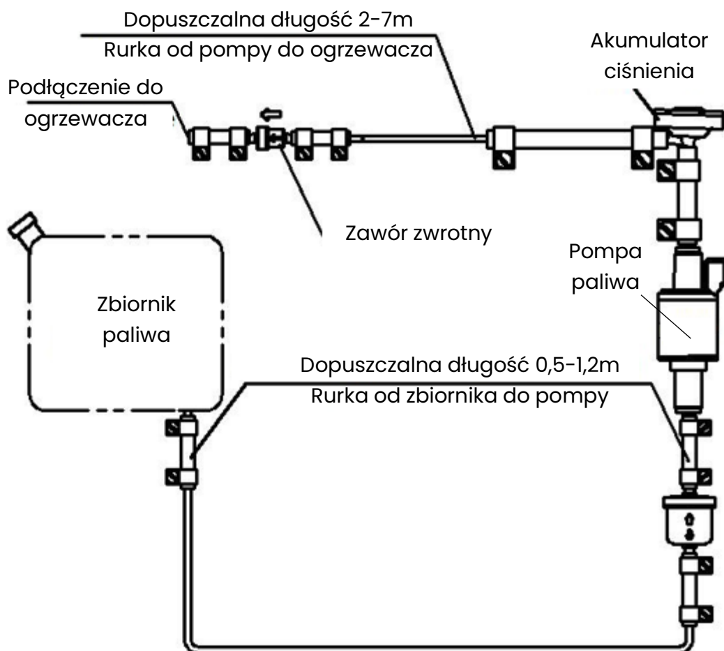
Rysunek 13 – Schemat podłączenia układu paliwowego.
