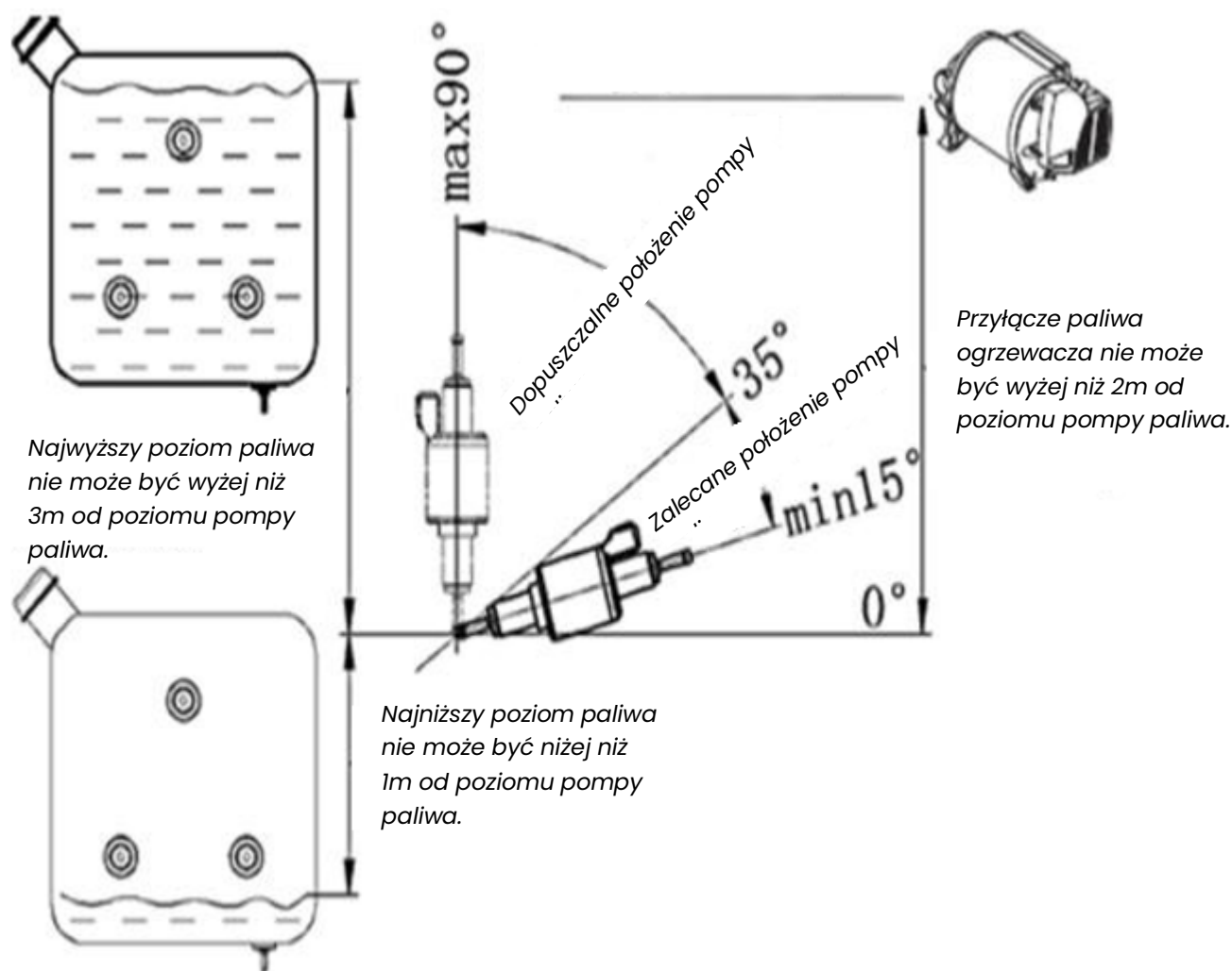
Rysunek 14 –Dopuszczalne położenie pompy paliwa.
