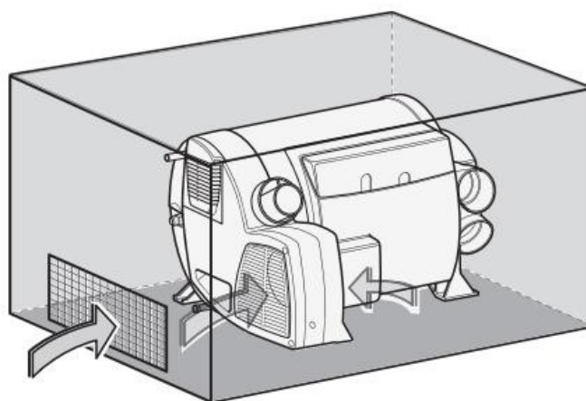
Rysunek 10 – Pobór powietrza do ogrzewania pomieszczenia
