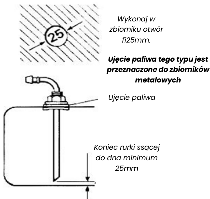
Rysunek 17 –Sposób montażu ujęcia paliwa w zbiorniku pojazdu.
